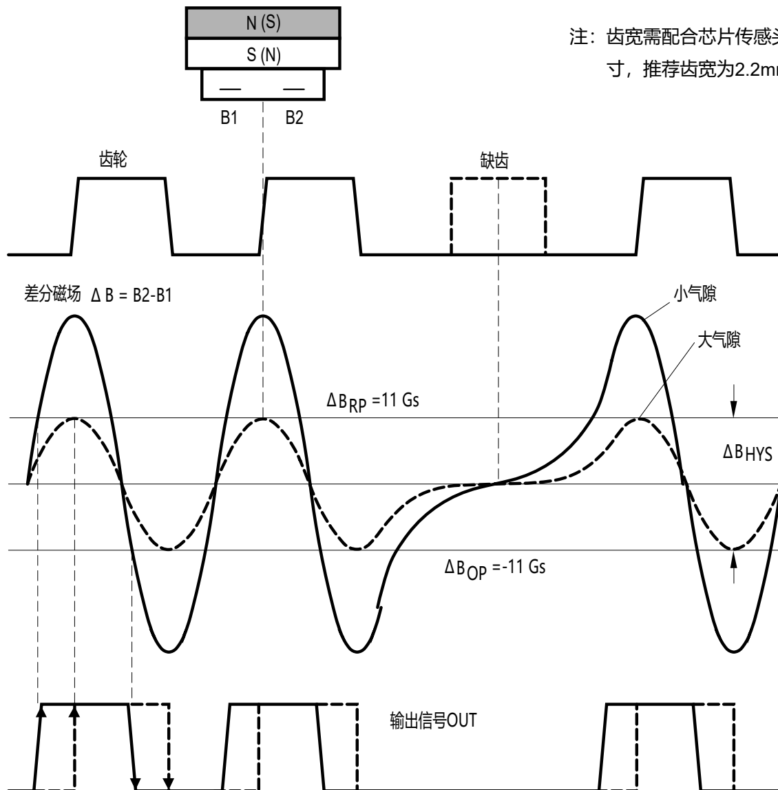
图 2, GH1922 做为齿轮传感器应用时的基本工作原理
