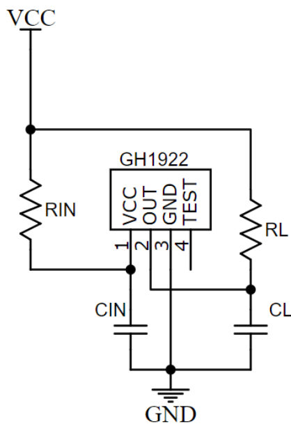
(A) 稳定电源下的应用
