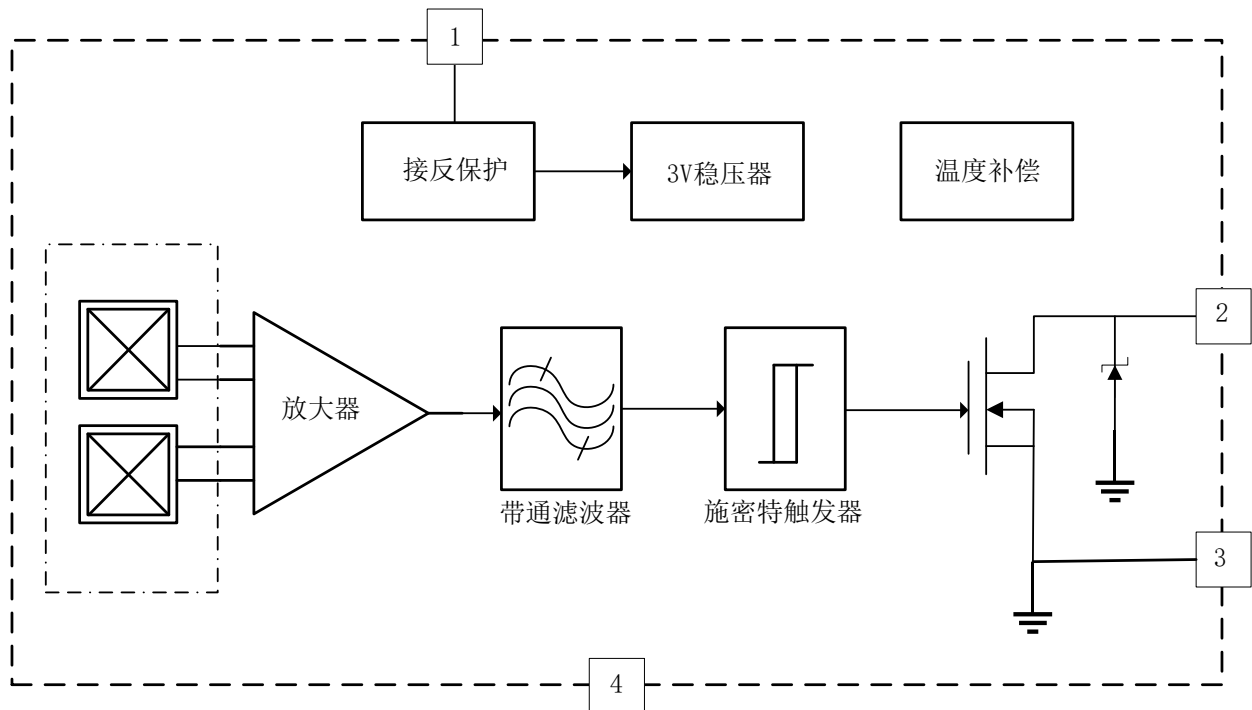
图 1, GH1922内部功能框图
